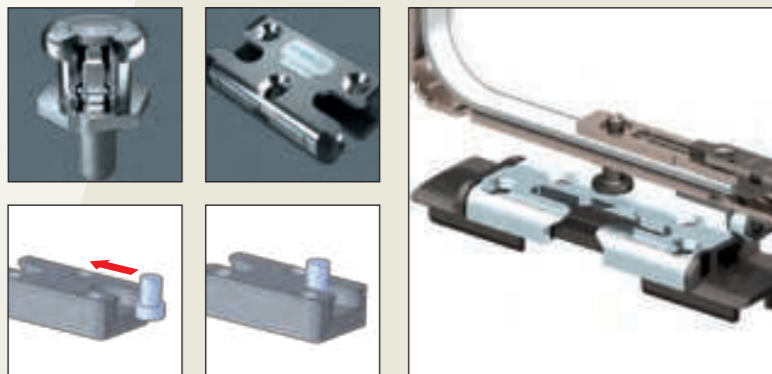
Rouleau KOPIBO et gâche de sécurité
